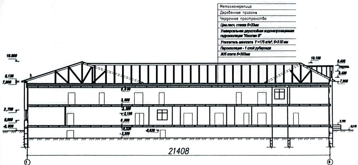
Разрез 1-1
