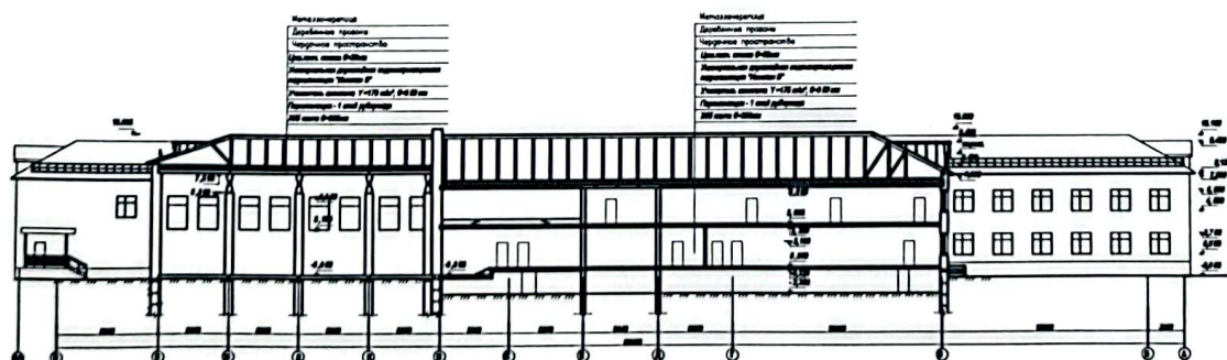
Разрез 2-2
